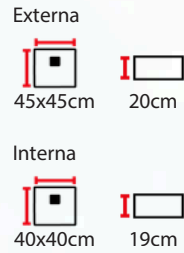
Cuba Inox Lux 500 Gold Escovado Cód: 311/002/002
